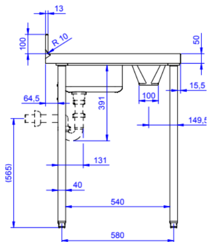
Sivulta
