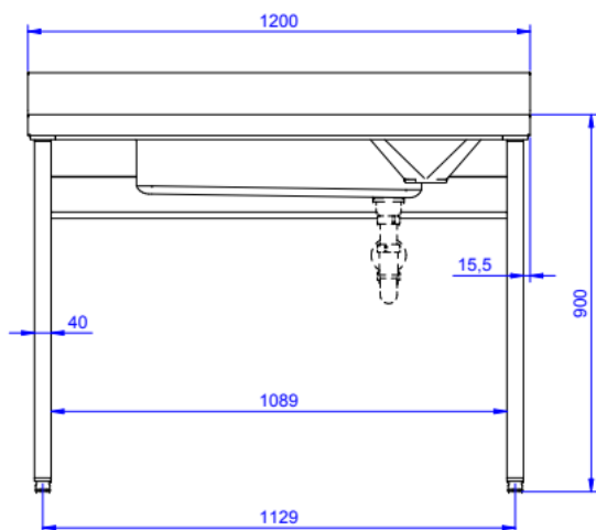
Edestä
